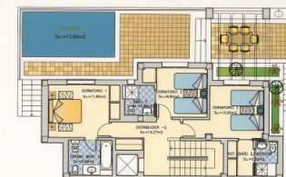
PLANTA -2 SUPERFICIE CONSTRUIDA SOBRE INCLINADO: 16,71m 2 SUPERFICIE CONSTRUIDA EN TERAPIANO: 116,49m 2
