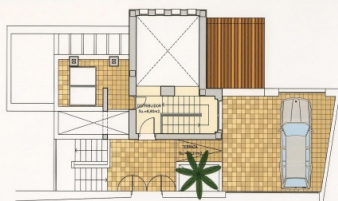
PLANTA DE ACCESO SUPERFICIE CONSTRUIDA: 12,14m 2
